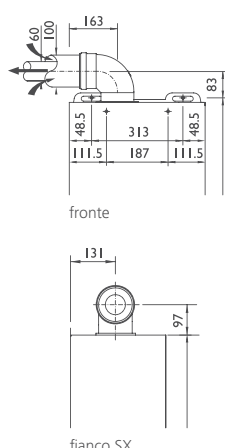
KIT K sistema coassiale orizzontale Ø 60/100
